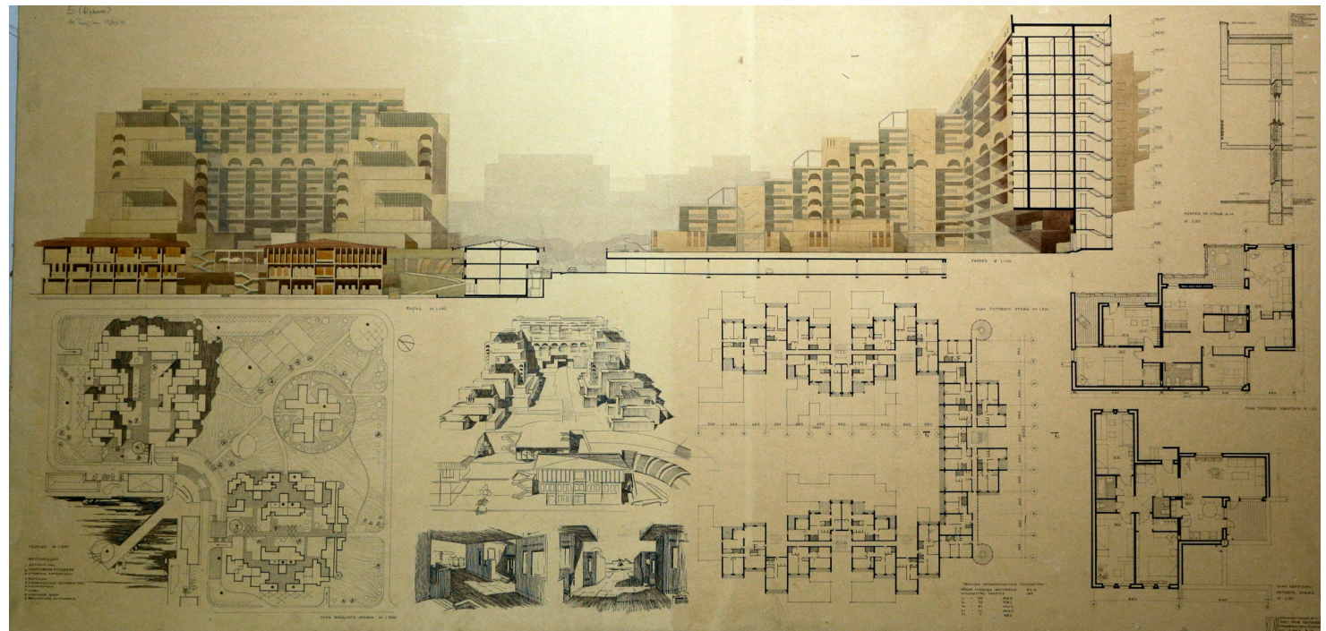
Олександр ДУМА Багатоповерховий житловий будинок Курсова робота, IV курс 1991 рік Керівник проекту проф. ЧМУТІНА Н.Б. Консультант доц. РОЗЕНБЕРГ В.А.
