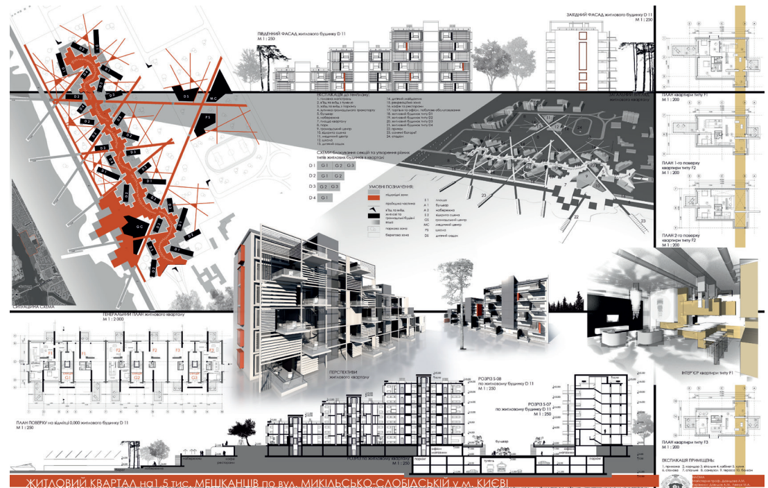
ЖИТЛОВИЙ КВАРТАЛ на 1,5 тис. мешканців по вул. МИКІЛЬСЬКО-СЛОБІДСЬКІЙ у м. КИЄВІ.
