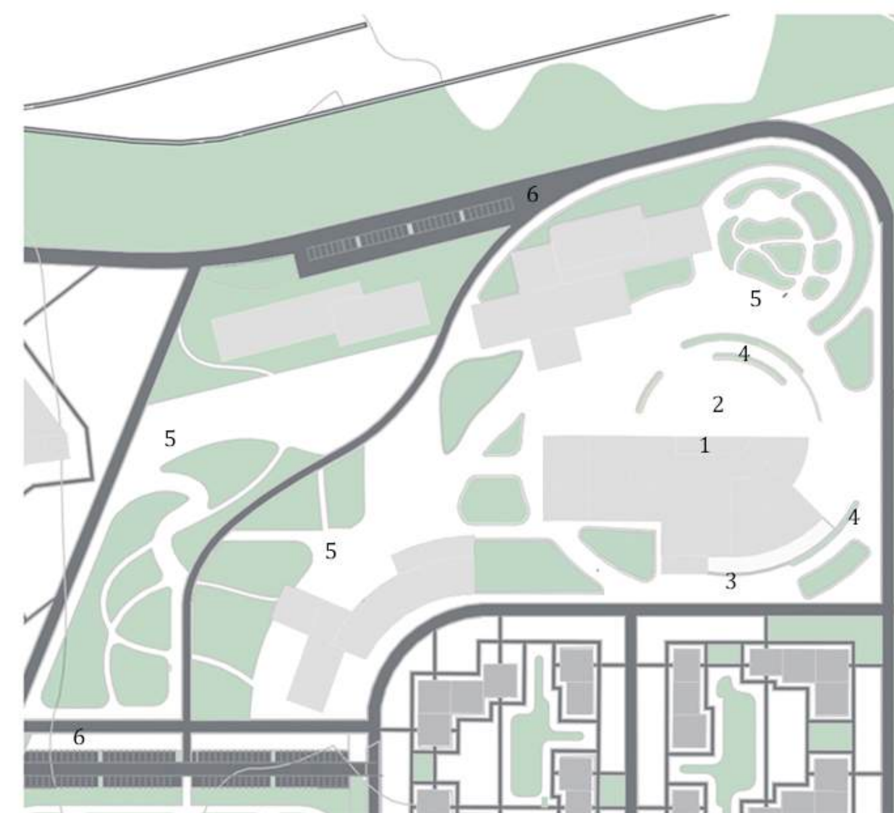
ГЕНЕРАЛЬНИЙ ПЛАН ДІЛЯНКИ 1:1000
