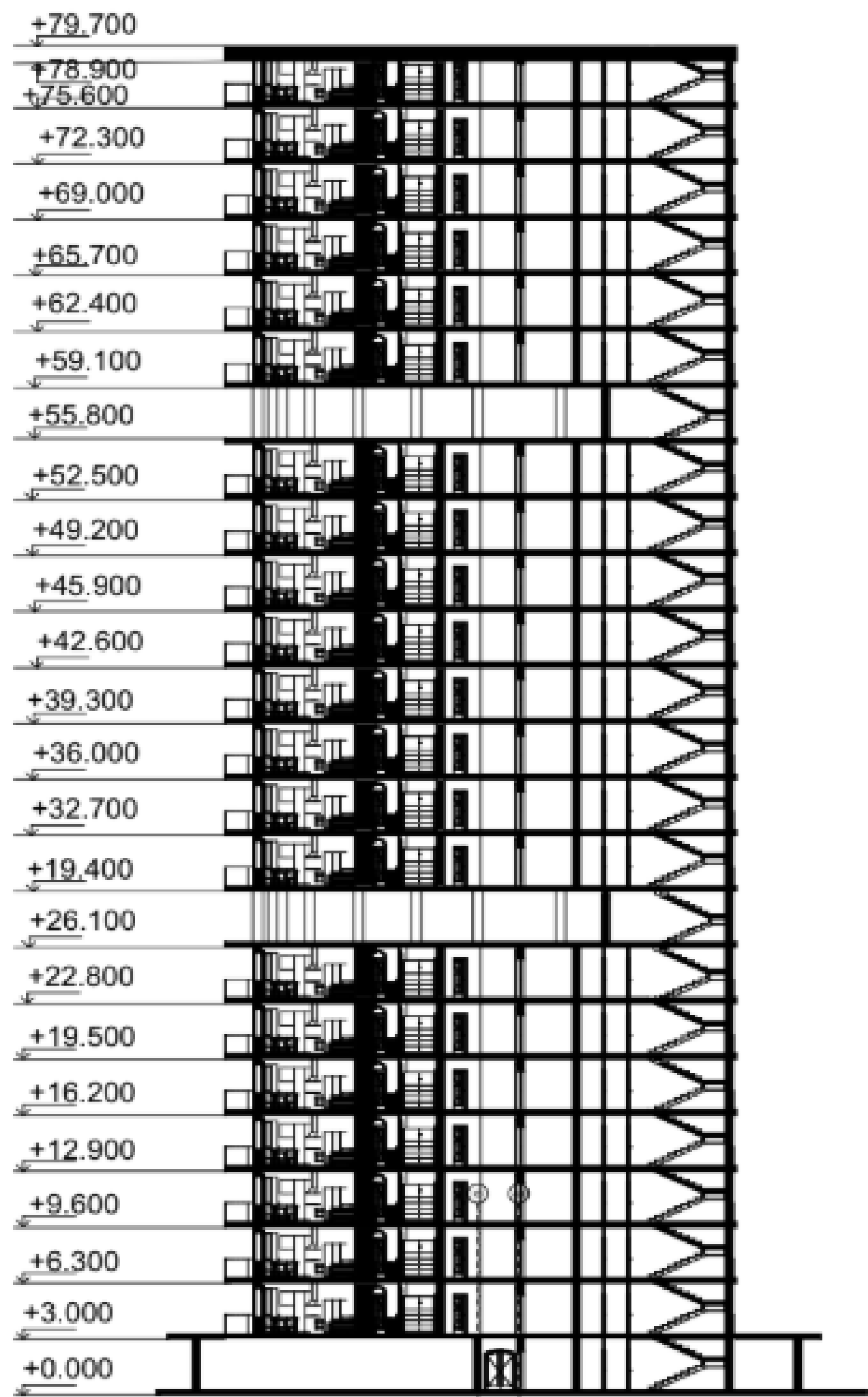
Розріз 1-1
