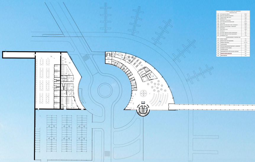
ПЛАН НА ВІДМІТЦІ \pm 0.000 М 1:300
