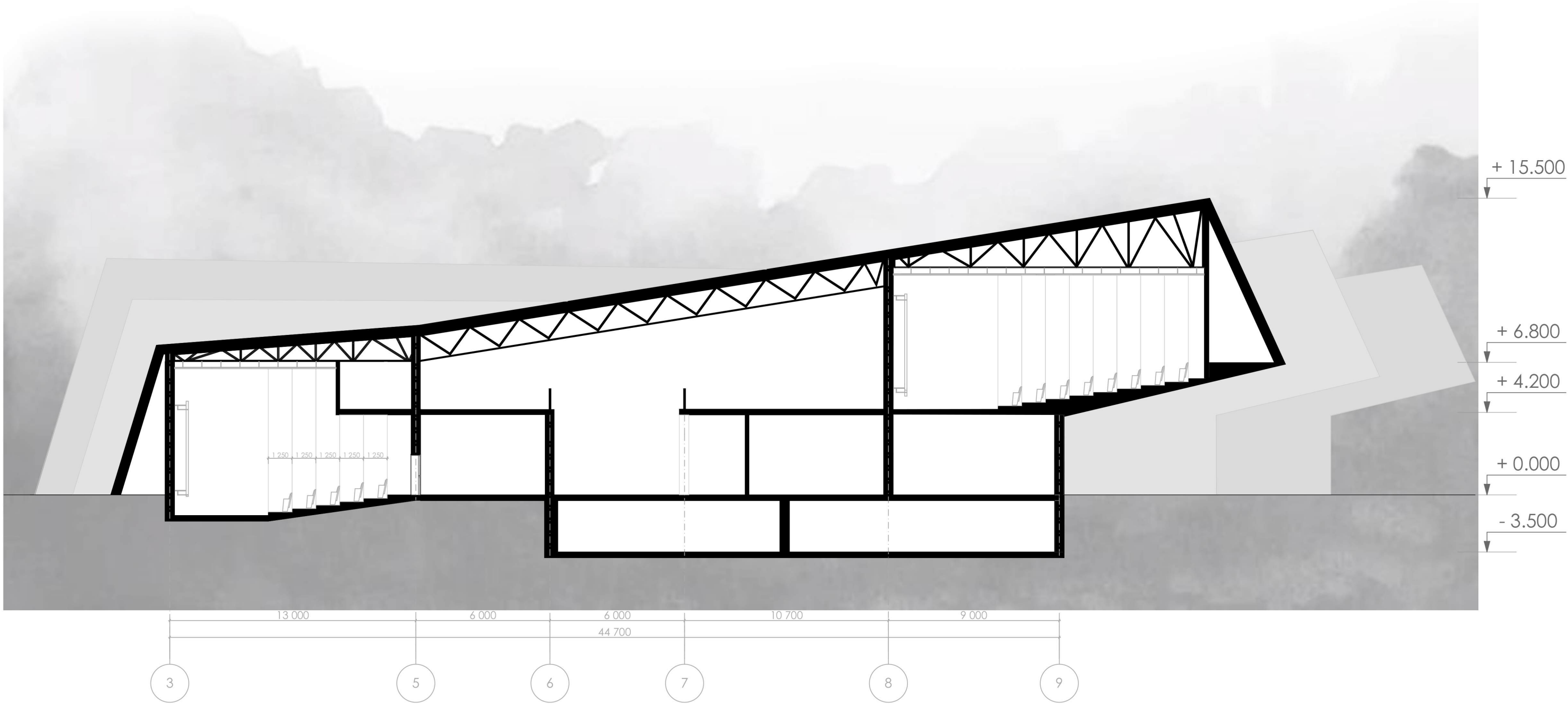
Розріз 1-1 М 1:200
