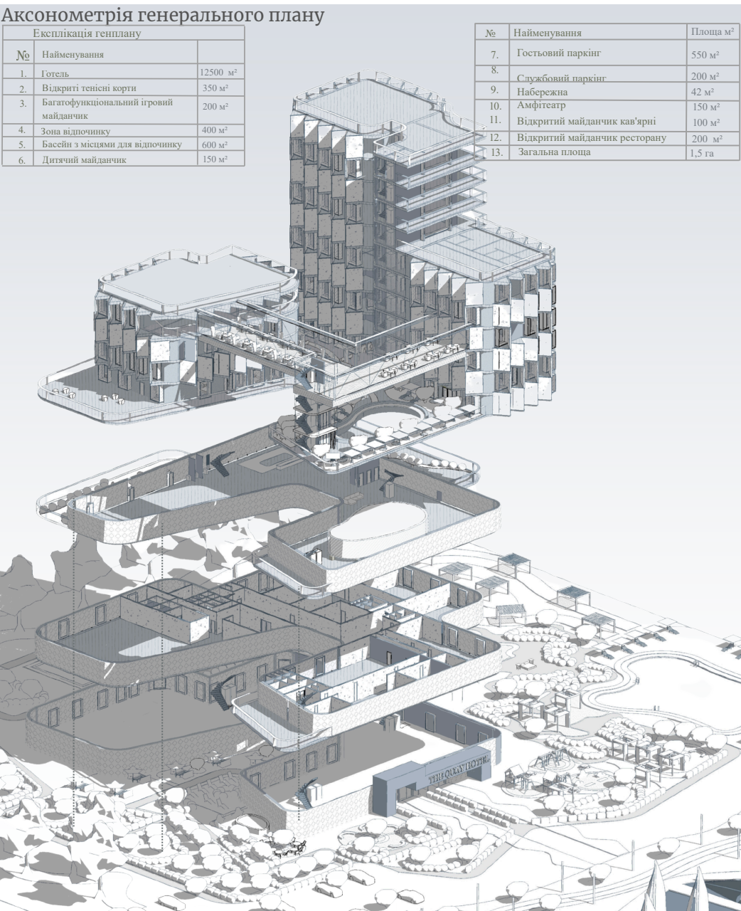
Аксонометрія генерального плану
