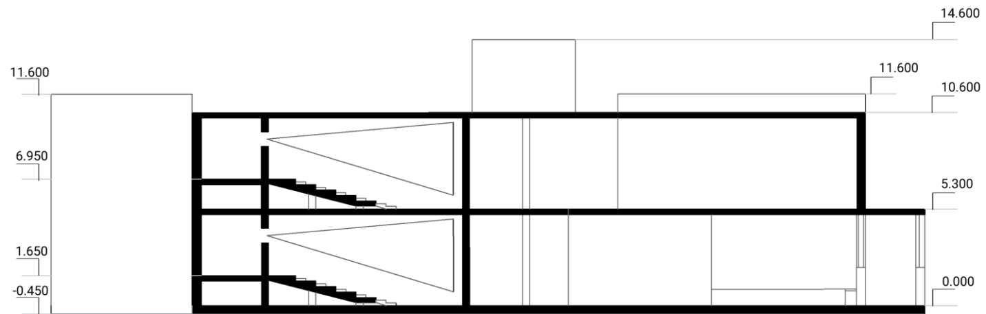
Розріз 1-1
