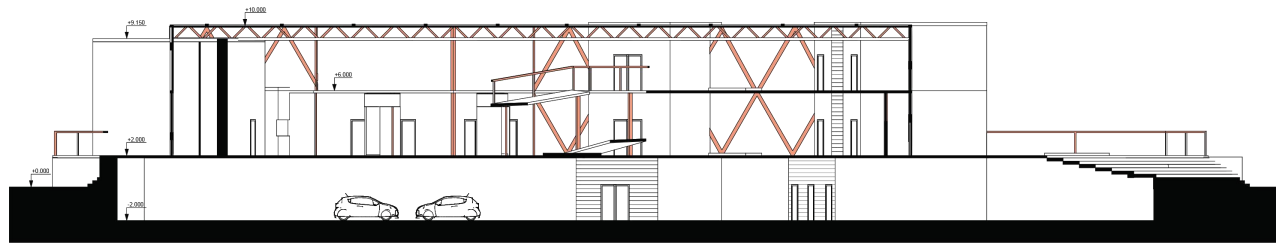
Розріз 1-1
