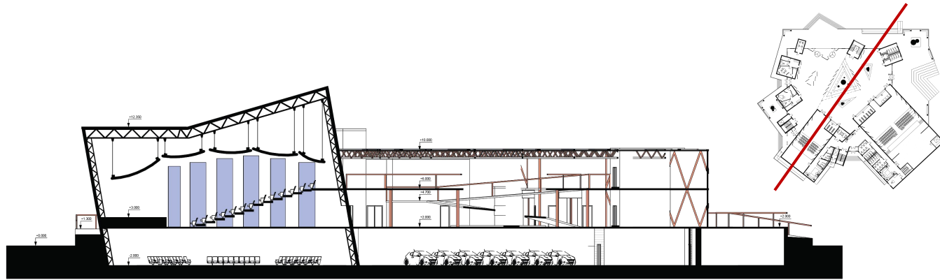
Розріз 2-2
