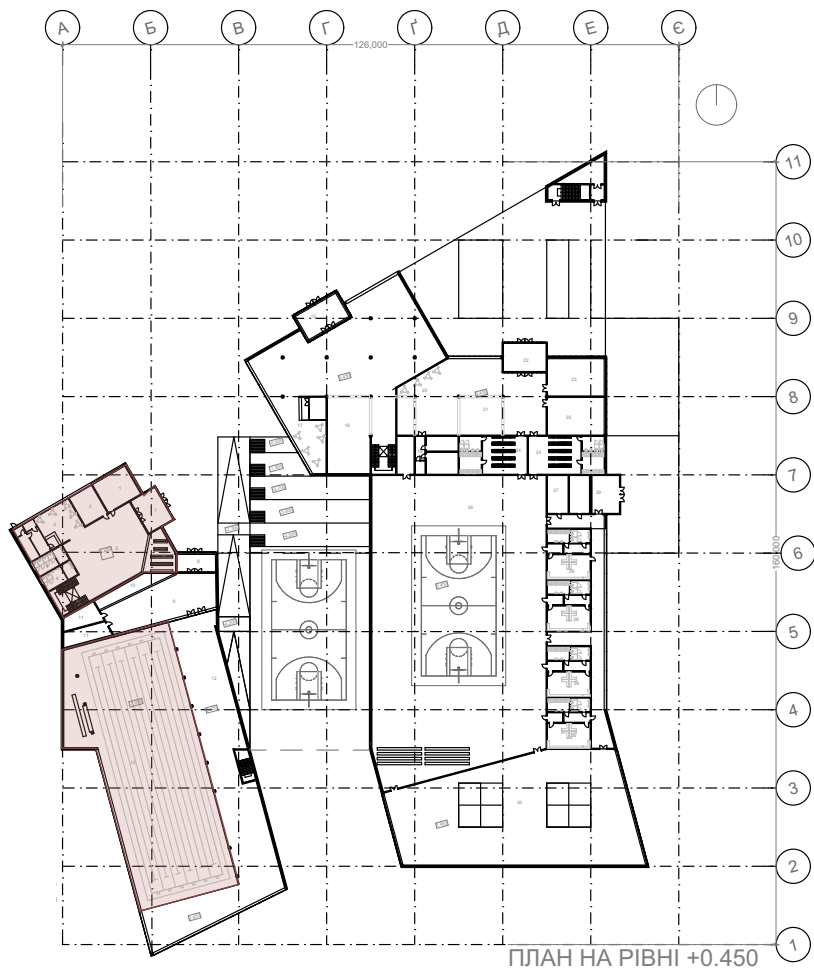
ПЛАН НА РІВНІ +0.450
