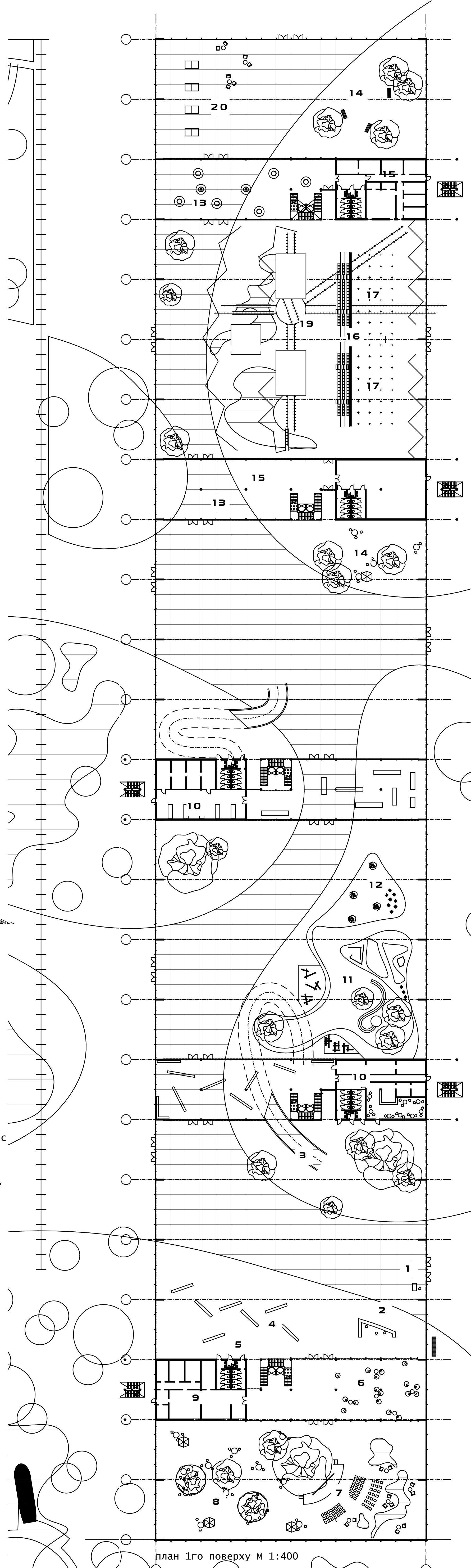
план 1го поверху М 1:400
