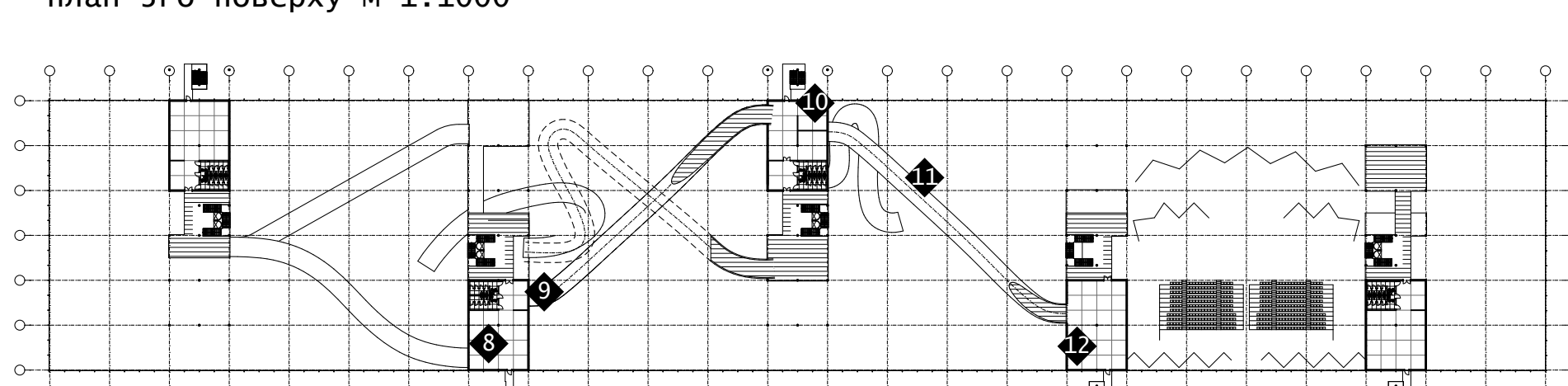
план 4го поверху М 1:1000
