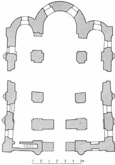
Іл. 2. Церква Успіння Богородиці Пирогошії на Подолі в Києві. План (І. Моргілевський). [8]
